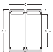
RNA69 (øFw ≥ 40 mm)
