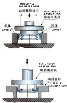
骨架油封不正确的组装 INCORRECT ASSEMBLING
