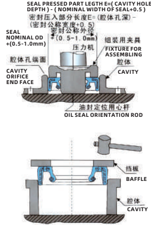
骨架油封的正确组装 CORRECT ASSEMBLING
