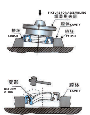
骨架油封不正确的组装 INCORRECT ASSEMBLING
