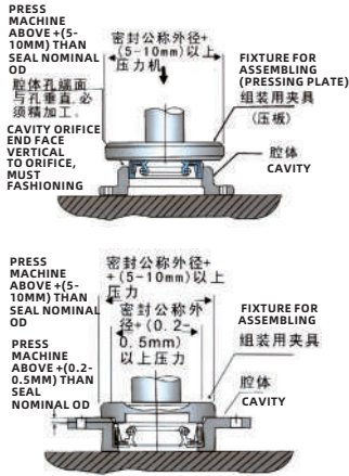
骨架油封的正确组装 CORRECT ASSEMBLING
