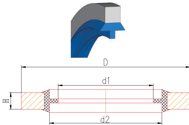
自定心镀锌 USIT-Ring I SF
