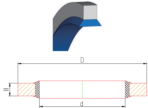
JB982-77国标 B型 USIT-Ring I
